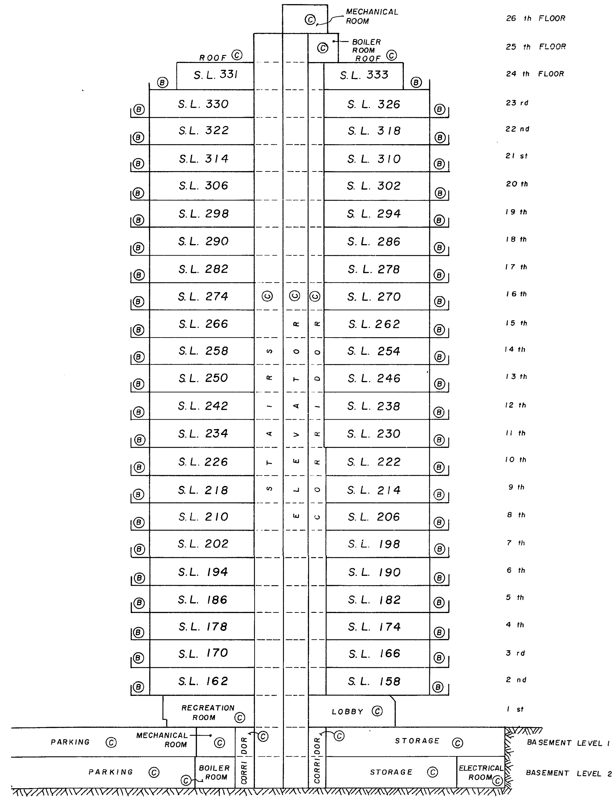
SECTION B - B'
